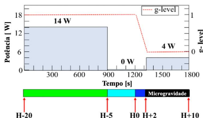
Fig. 9. Procedimento de teste do LHP plano miniaturizado, simulando voo suborbital [6].
