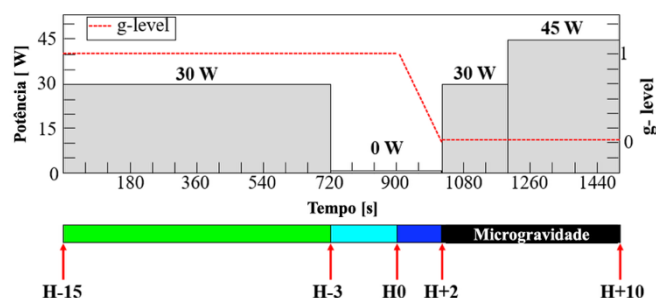
Fig. 8. Procedimento de teste do LHP tubular simulando voo suborbital.
