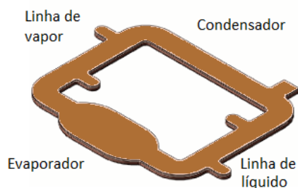
Fig. 7. LHP plano miniaturizado.
