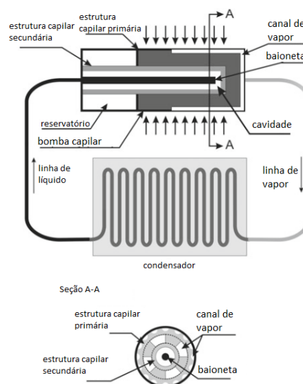
Fig. 1. Esquema do princípio de funcionamento de um tubo de calor em circuito.
