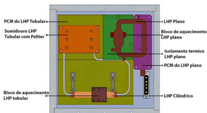
Fig. 5. Esquemático da seção do experimento térmico.
