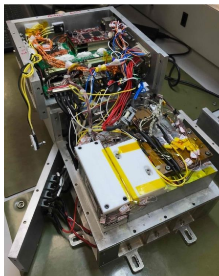
Fig. 3. Vista da plataforma experimental MPM-A.
