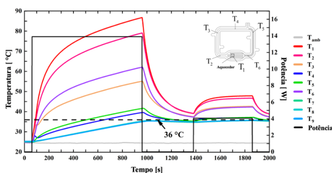
Fig. 10. Distribuição de temperaturas do LHP plano miniaturizado [3].
