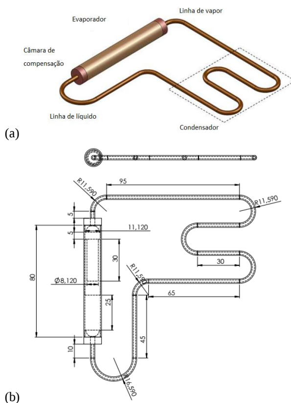
Fig. 6. LHP tubular (a) seções (b) dimensões.
